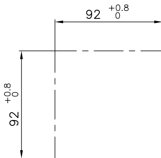
Schalttafel Ausschnitt M1:2
