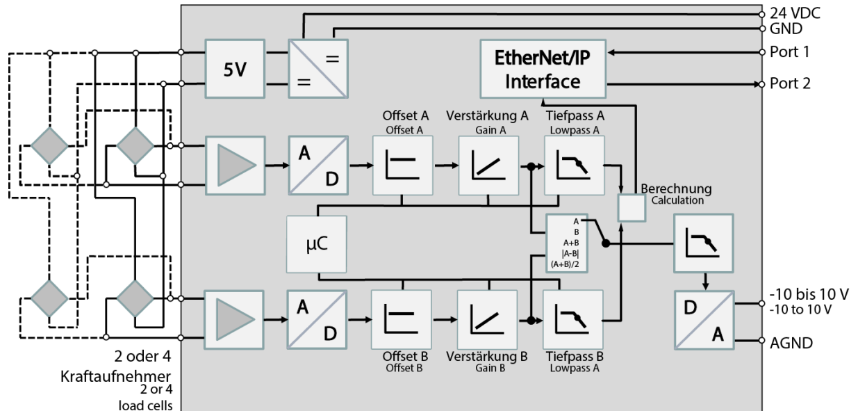
Abbildung 1: Blockschaubild EMGZ492.EIP
