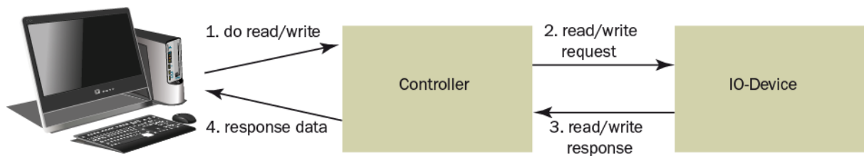
Abbildung 8: Read- / Write-Zyklus
