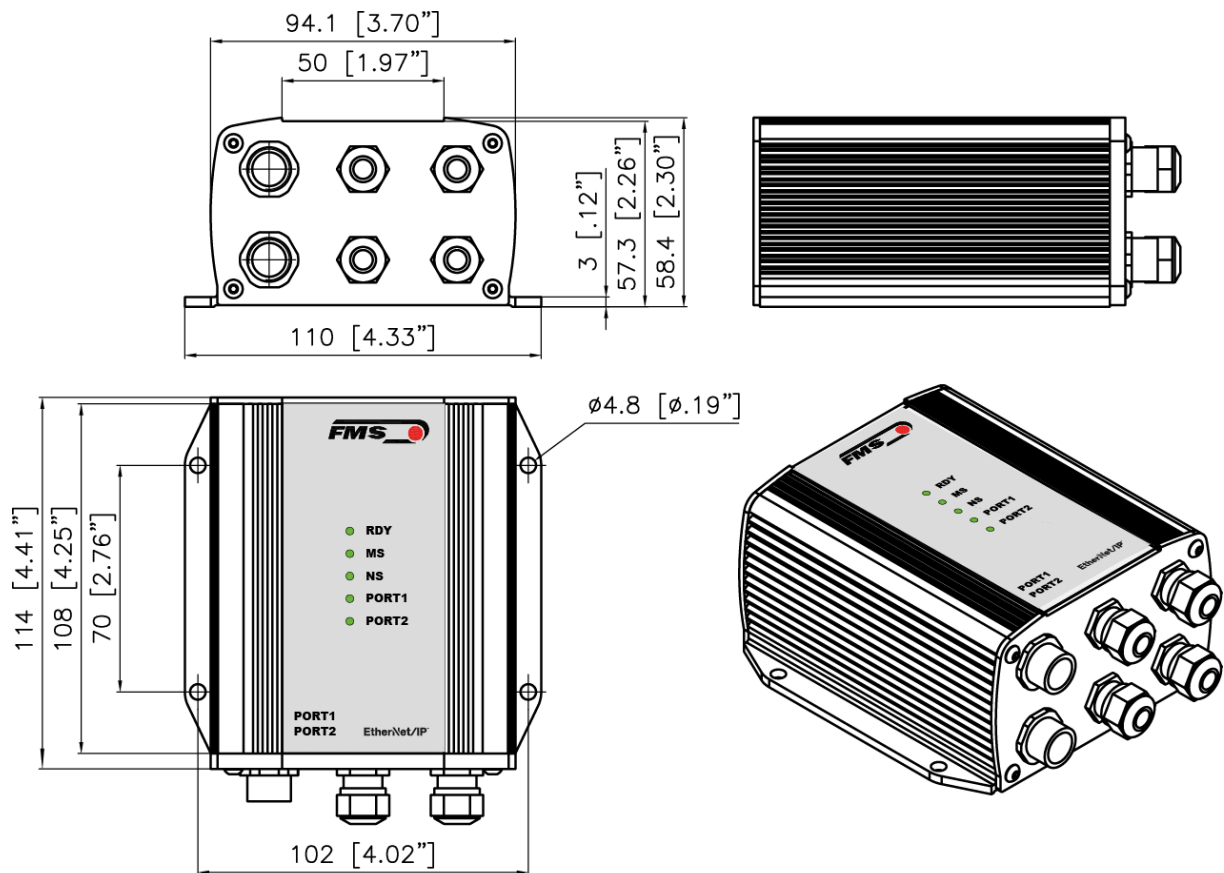
Abbildung 16: EMGZ491.W.EIP Gehäuse für Wandmontage
