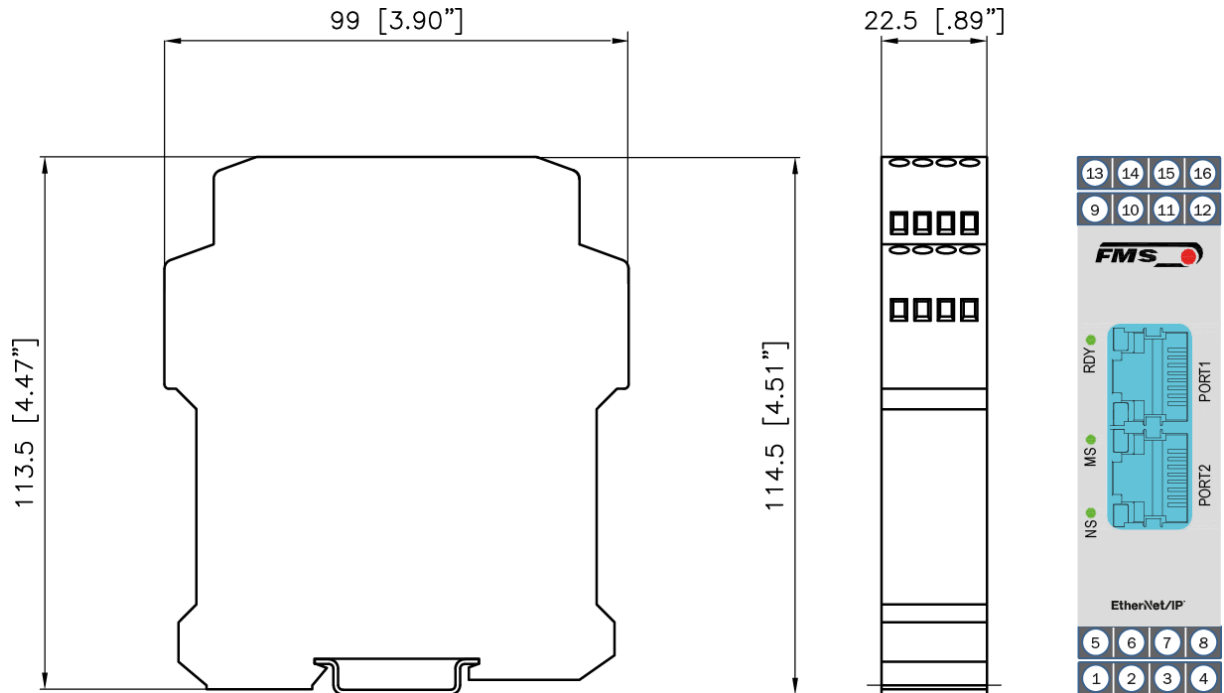
Abbildung 15: EMGZ491.R.EIP Gehäuse für DIN-Schiennenmontage EMGZ491_EIP_BA_Manual.ai
